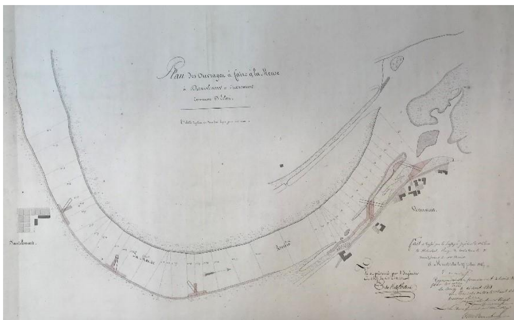
Plan voor oeverbeschermingswerken bij Visserweert (1818), HCL, Rijkswaterstaat, inv.nr. 1739
