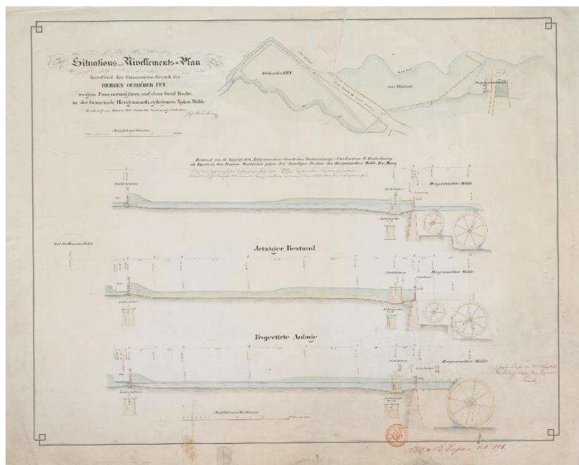
Tekening van voorgenomen werken aan de molen van de gebroeders Fey te Hergenrath aan de Geul, Landesarchiv NRW, Abteilung Rheinland.
